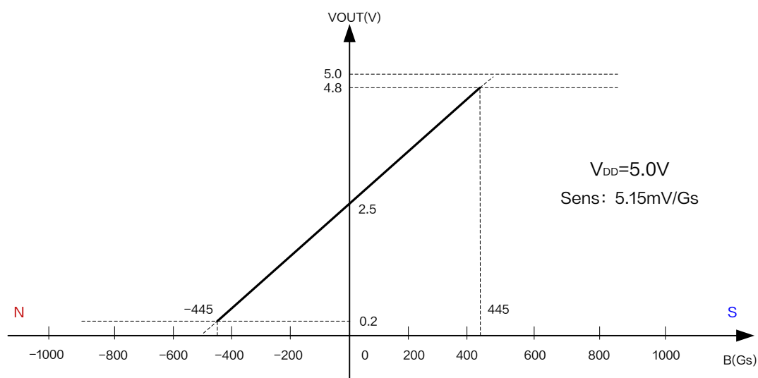
图 6.XL45T 输出特性曲线 ( V_{DD} = 5.0V )
