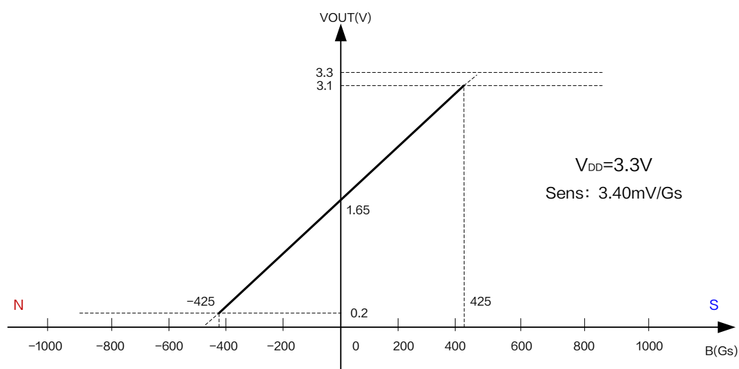
图 5.XL45T 输出特性曲线 ( V_{DD} = 3.3\text{V} )
