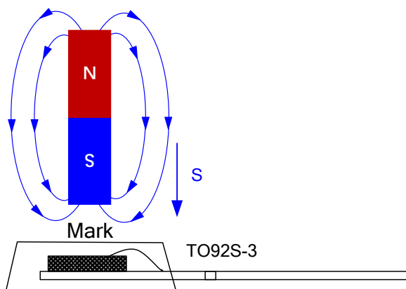
图 4.XL45T 测试示意图
