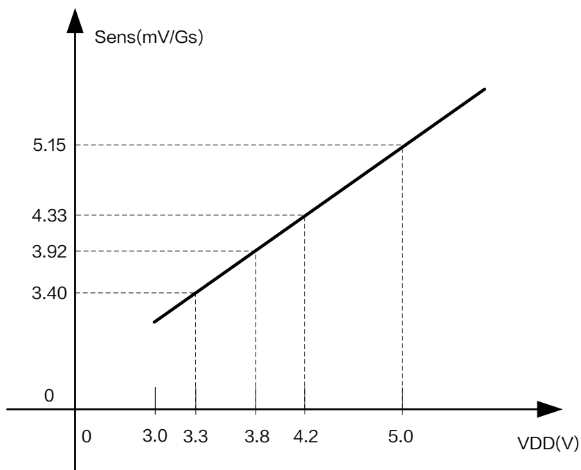
图 7.XL45T 灵敏度线性曲线
