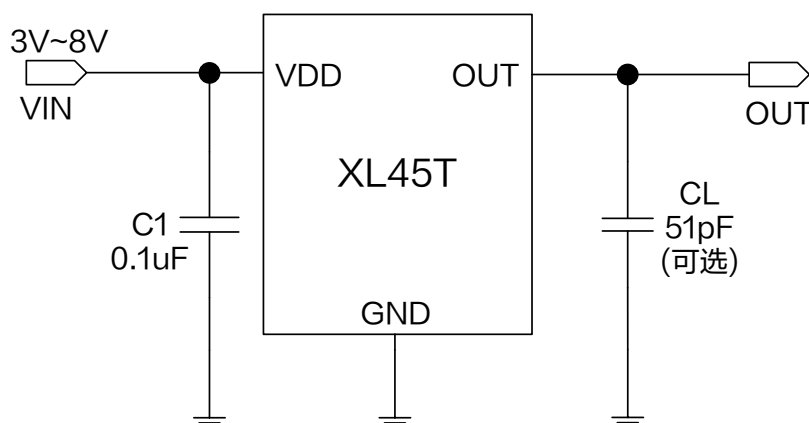
图 1.XL45T 典型应用示意图
