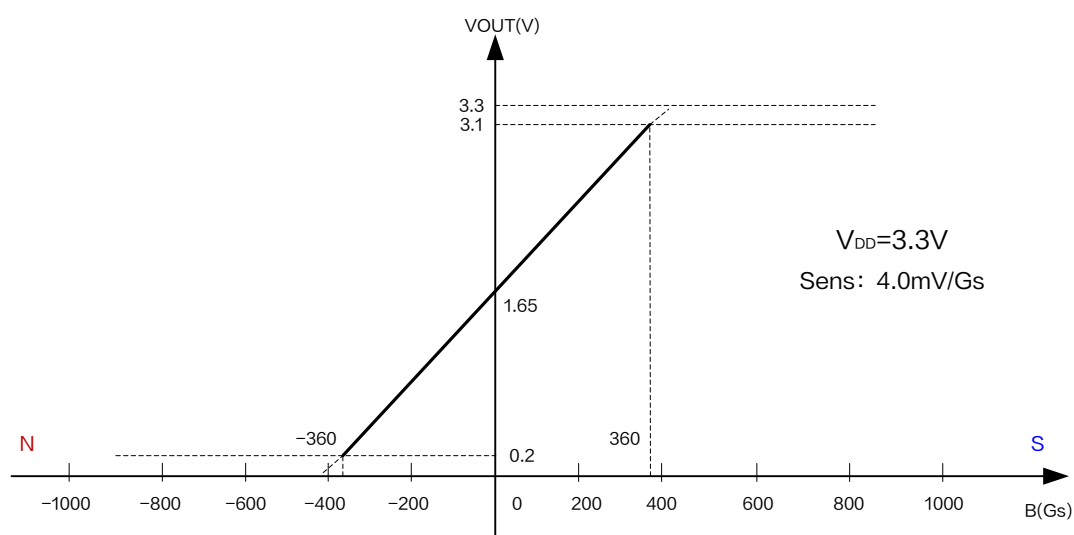
图 5.XL44T 输出特性曲线 ( V_{DD} = 3.3\text{V} )
