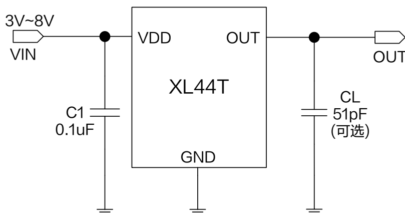
图 1.XL44T 典型应用示意图
