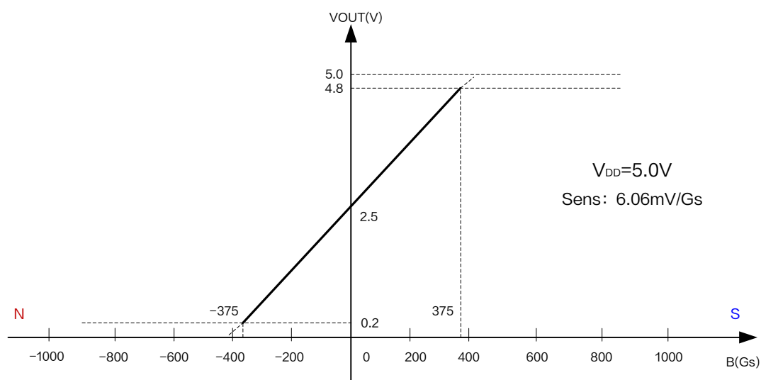
图 6.XL44T 输出特性曲线 ( V_{DD} = 5.0V )
