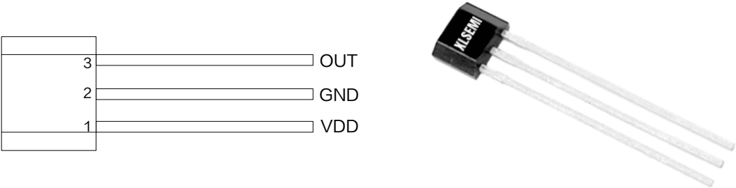
图 2.XL44T 引脚配置
