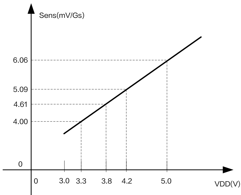
图 7.XL44T 灵敏度线性曲线
