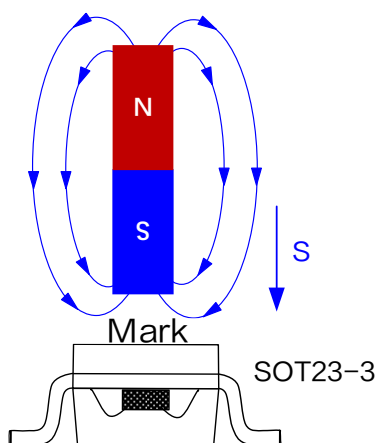
图 4.XL44B 测试示意图
