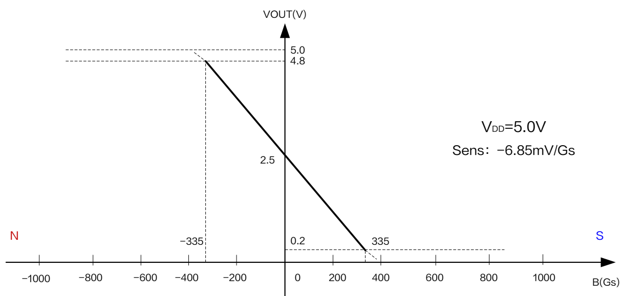
图 6.XL44B 输出特性曲线 ( V_{DD} = 5.0V )
