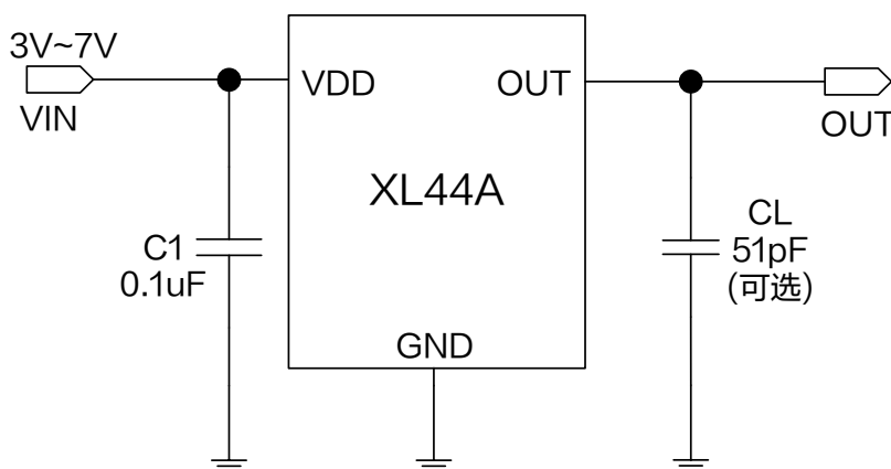
图 1.XL44A 典型应用示意图
