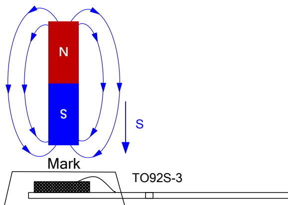
图 4.XL44A 测试示意图
