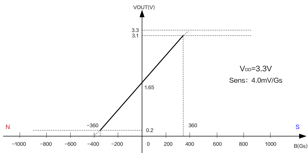
图 5.XL44A 输出特性曲线 ( V_{DD} = 3.3\text{V} )
