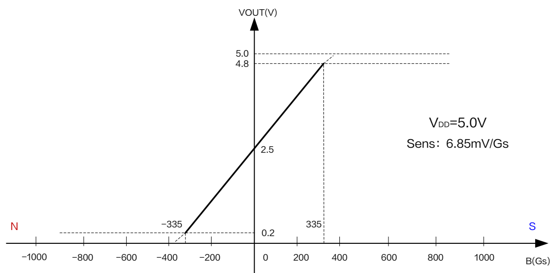
图 6.XL44A 输出特性曲线 ( V_{DD} = 5.0V )
