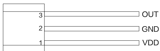
图 2.XL44A 引脚配置
