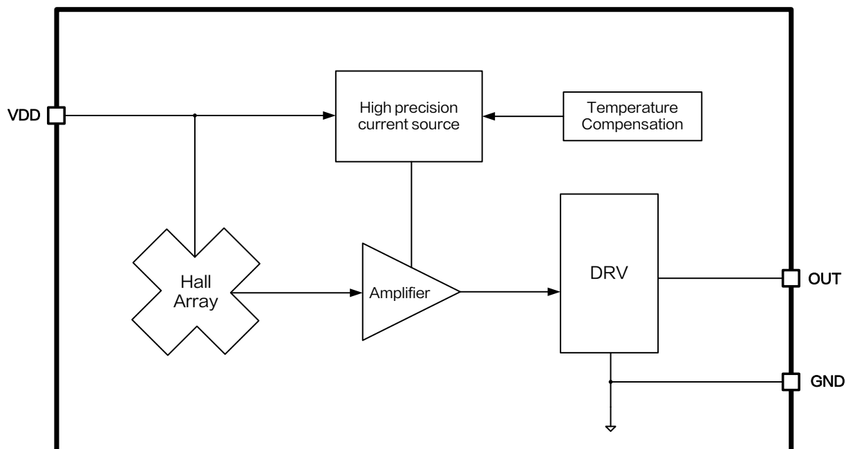
图 3.XL44A 功能方框图
