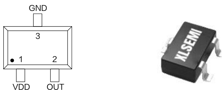
图 2.XL42Z 引脚配置
