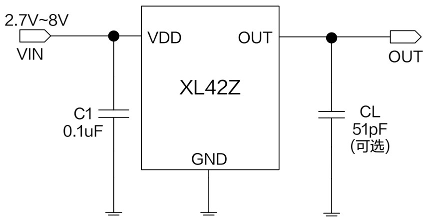
图 1.XL42Z 典型应用示意图
