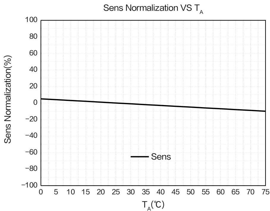
图 7.XL42Z 灵敏度随温度变化曲线 ( V_{DD} = 3.3V )
