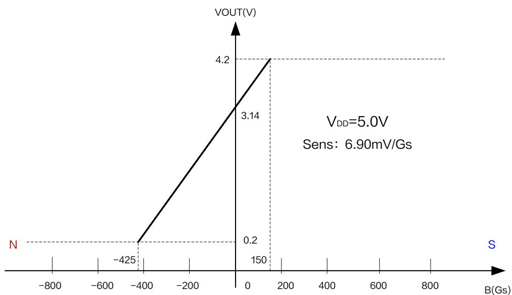
图 6.XL42Z 输出特性曲线 ( V_{DD} = 5.0V )
