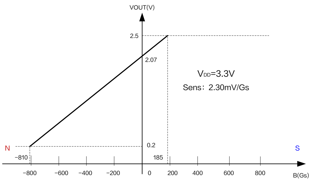
图 5.XL42Z 输出特性曲线 ( V_{DD} = 3.3V )
