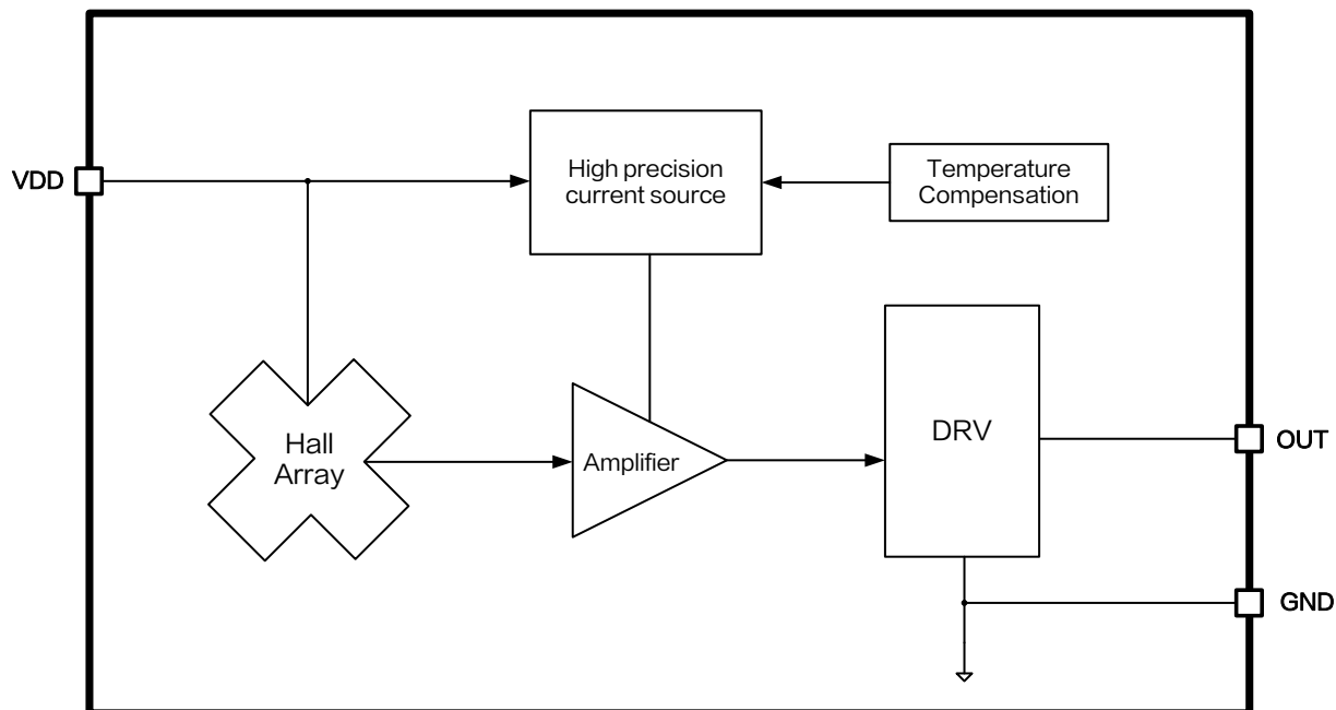
图 3.XL42X 功能方框图
