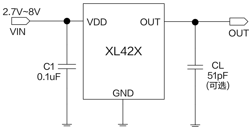
图 1.XL42X 典型应用示意图
