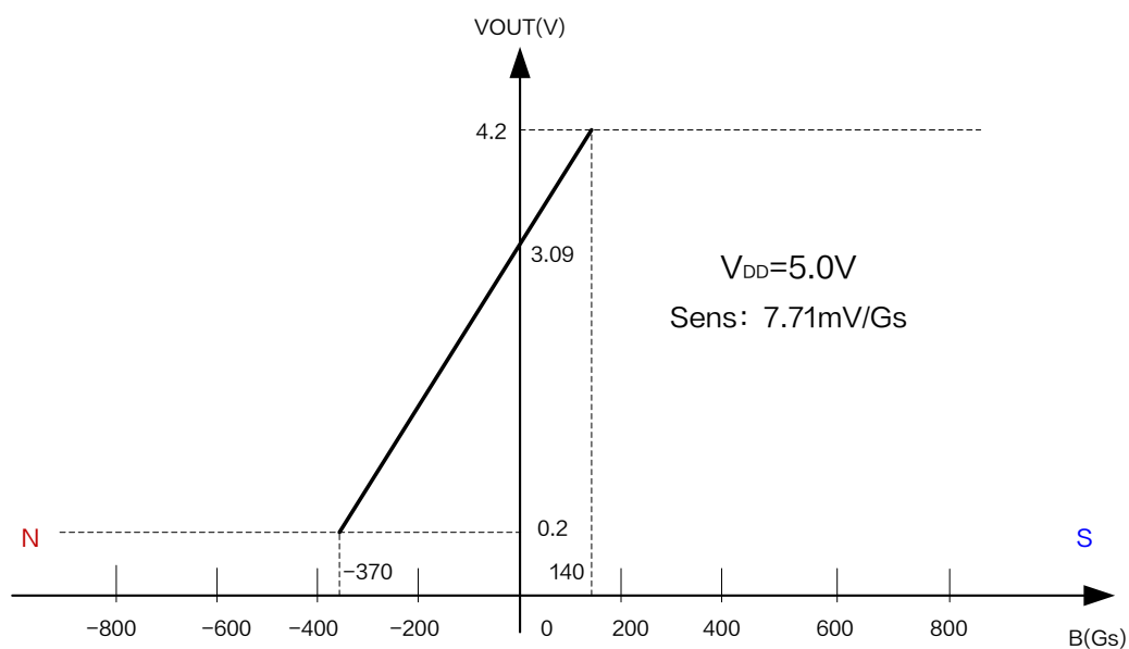
图 6.XL42X 输出特性曲线 ( V_{DD} = 5.0V )
