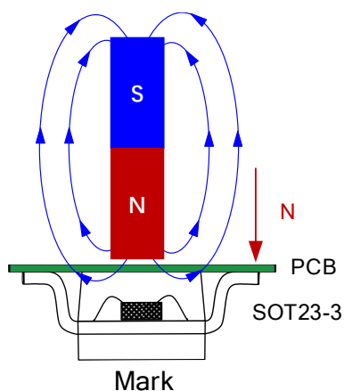
图 4.XL42X 应用图
