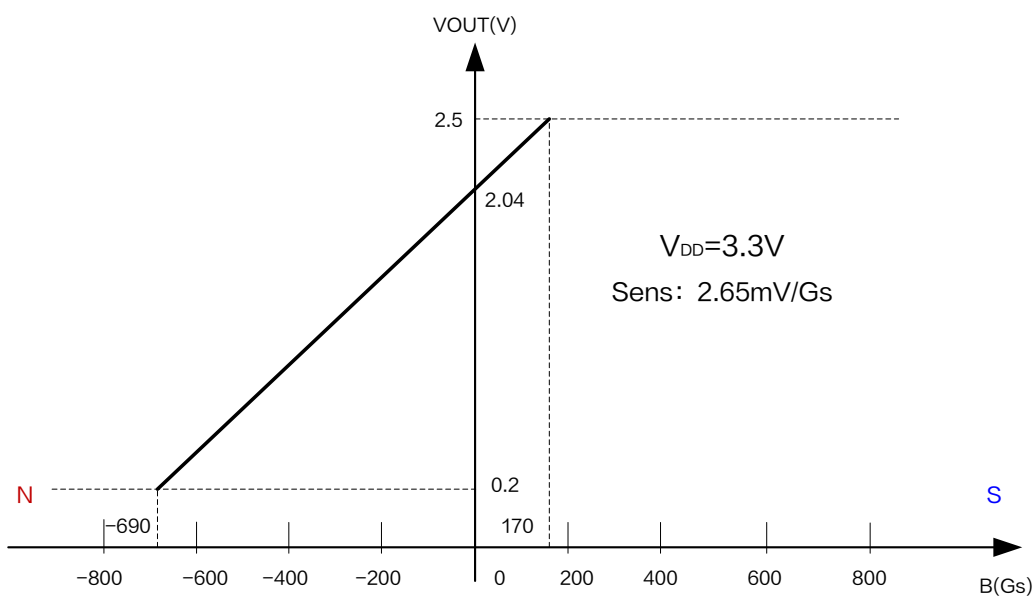
图 5.XL42X 输出特性曲线 ( V_{DD} = 3.3\text{V} )
