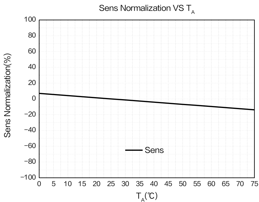
图 7.XL42X 灵敏度随温度变化曲线 ( V_{DD} = 3.3V )
