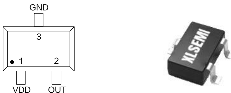
图 2.XL42X 引脚配置
