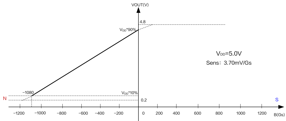
图 6.XL42K 输出特性曲线 ( V_{DD} = 5.0V )
