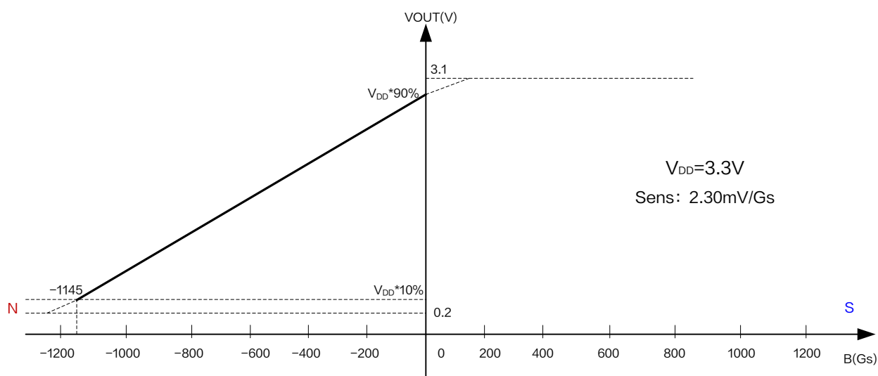
图 5.XL42K 输出特性曲线 ( V_{DD} = 3.3V )
