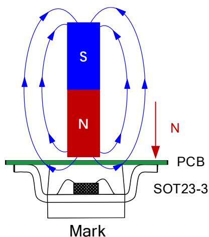
图 4.XL42K 应用图
