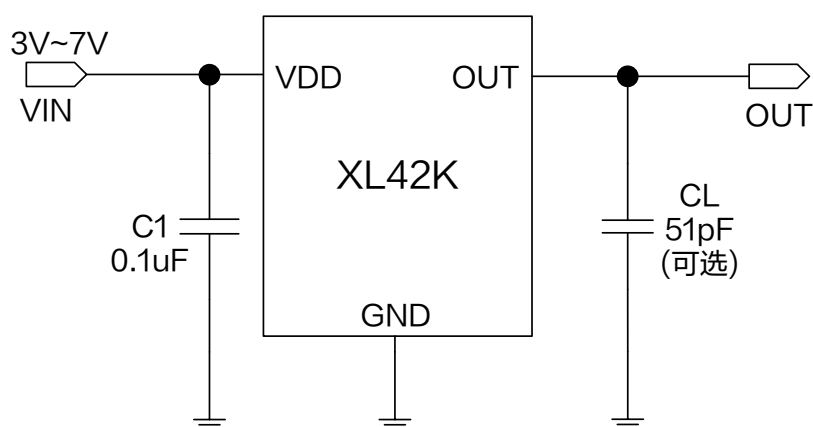
图 1.XL42K 典型应用示意图
