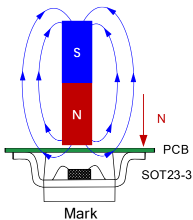
图 4.XL41Z 应用图
