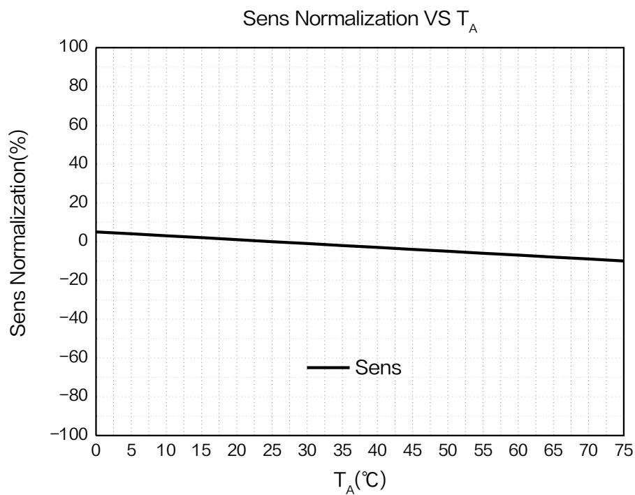
图 7.XL41Z 灵敏度随温度变化曲线 ( V_{DD} = 3.3V )
