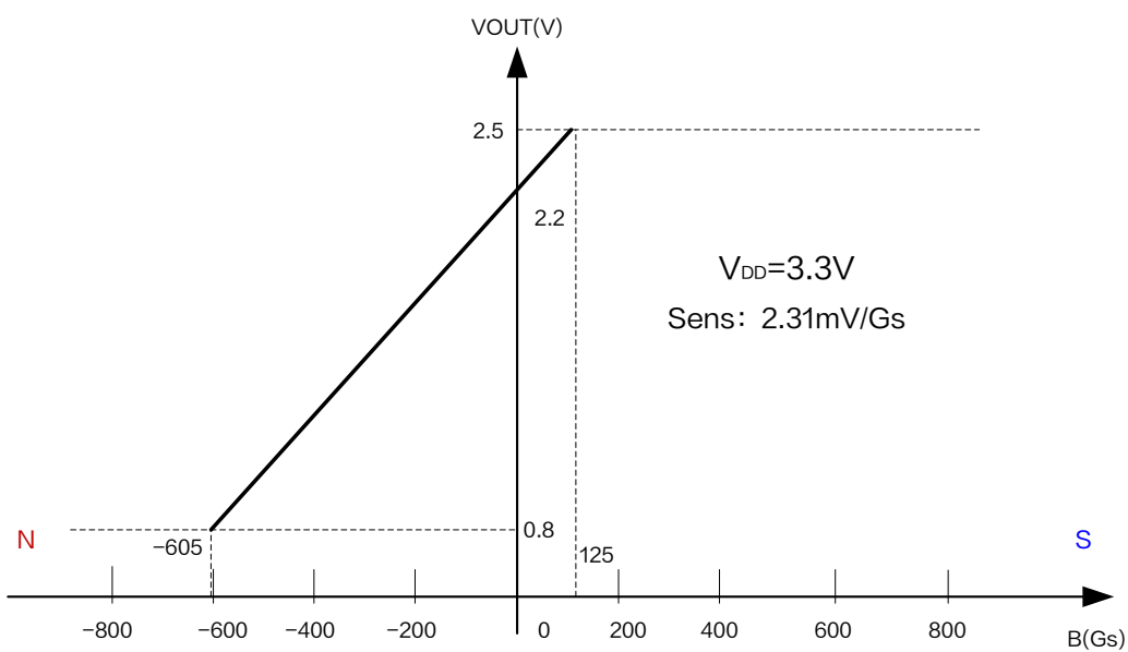
图 5.XL41Z 输出特性曲线 ( V_{DD} = 3.3V )
