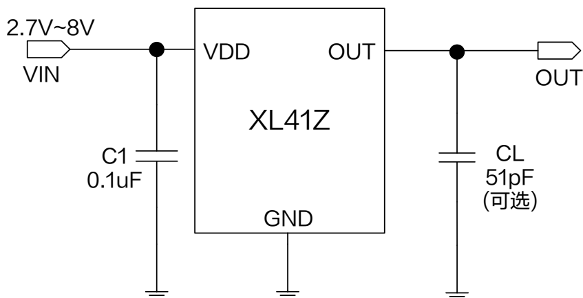
图 1.XL41Z 典型应用示意图
