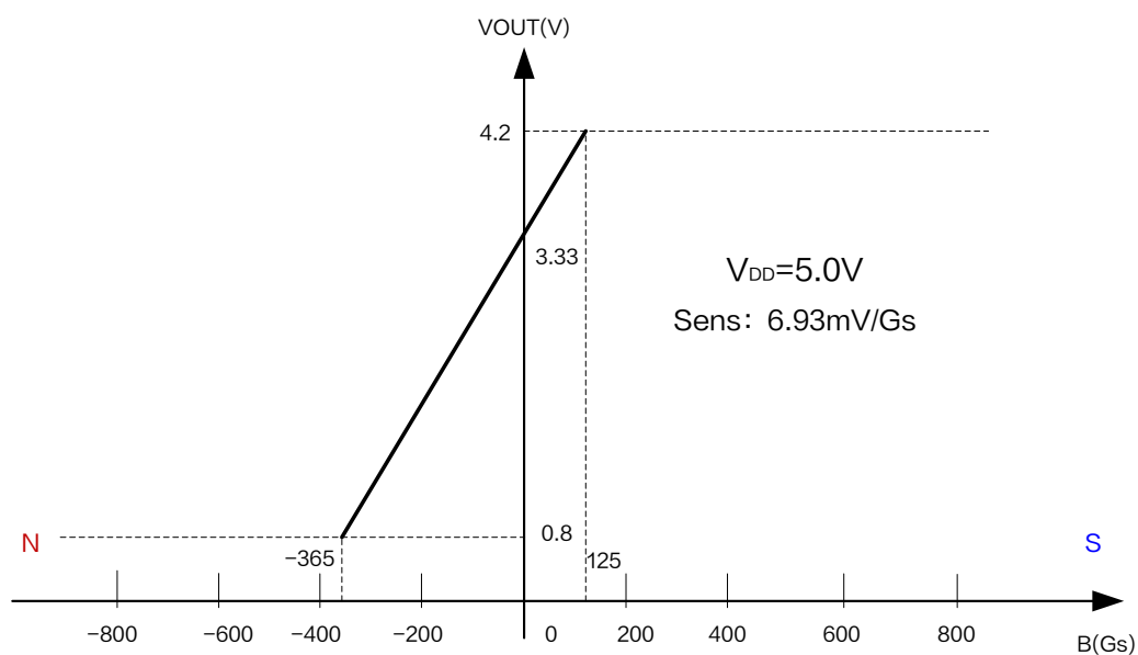
图 6.XL41Z 输出特性曲线 ( V_{DD} = 5.0V )
