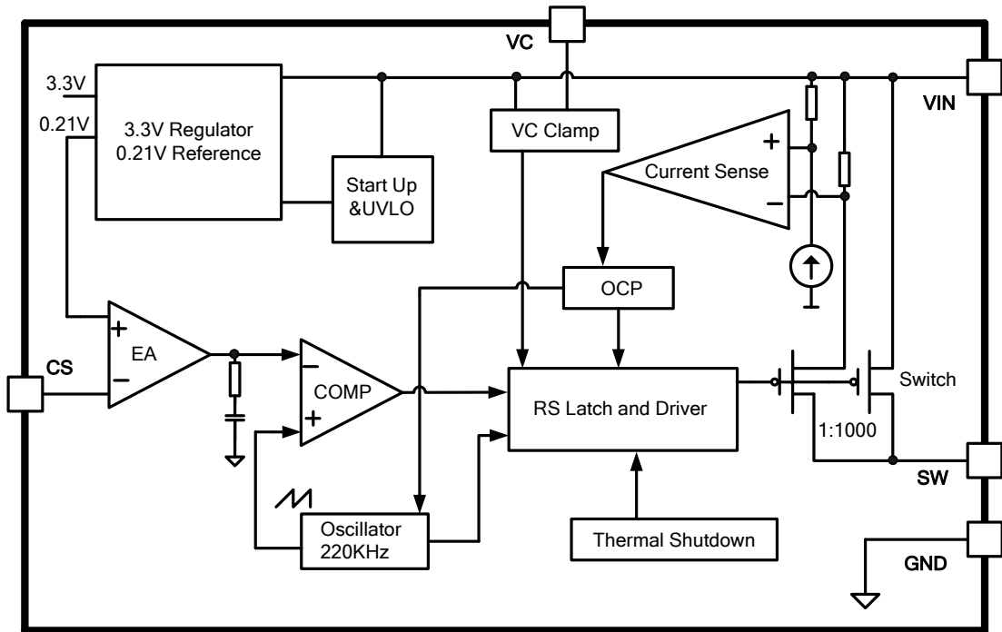
图 3. XL3005 方框图
