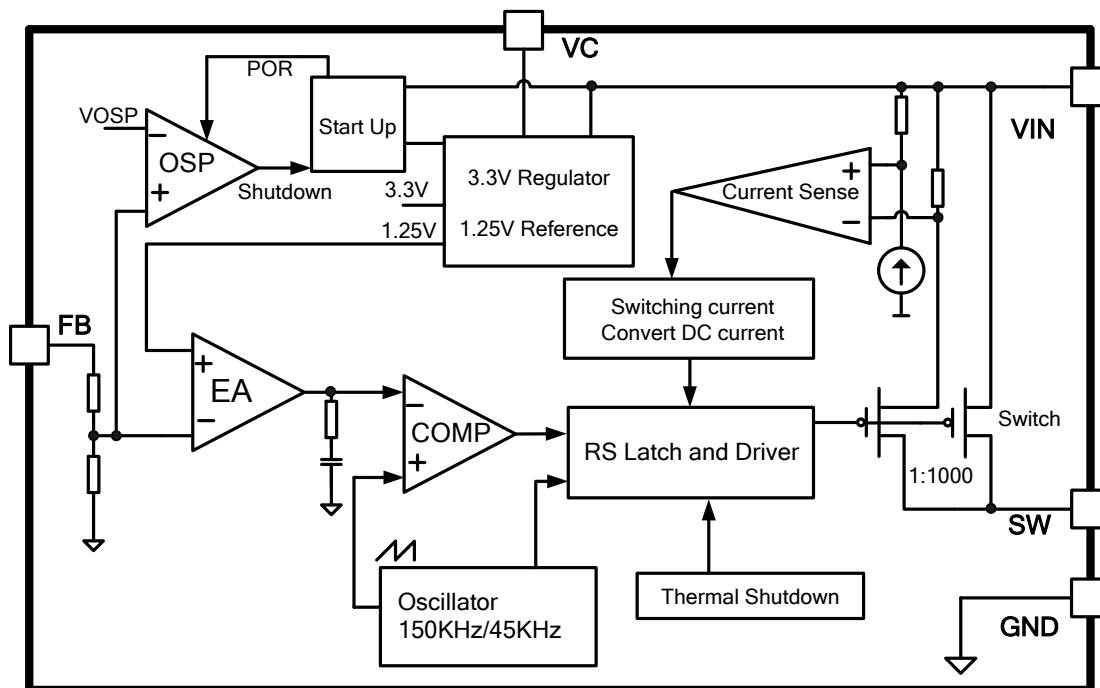
图 3. XL2011 方框图
